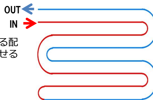
(送戻交互配管例)
