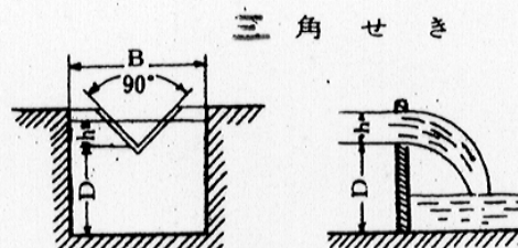
三 角 形 堰 TRIANGULAR WEIR
